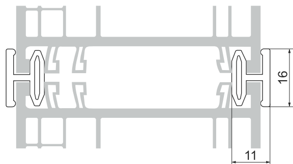
Рама GEALAN S 8000
